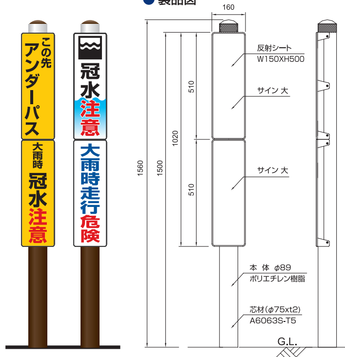
● 製品図
