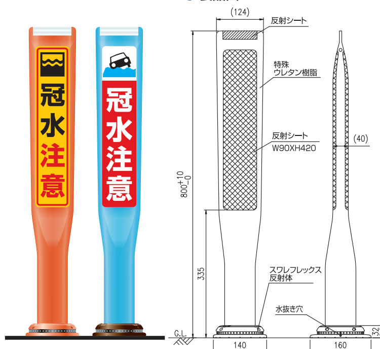
● 製品図
