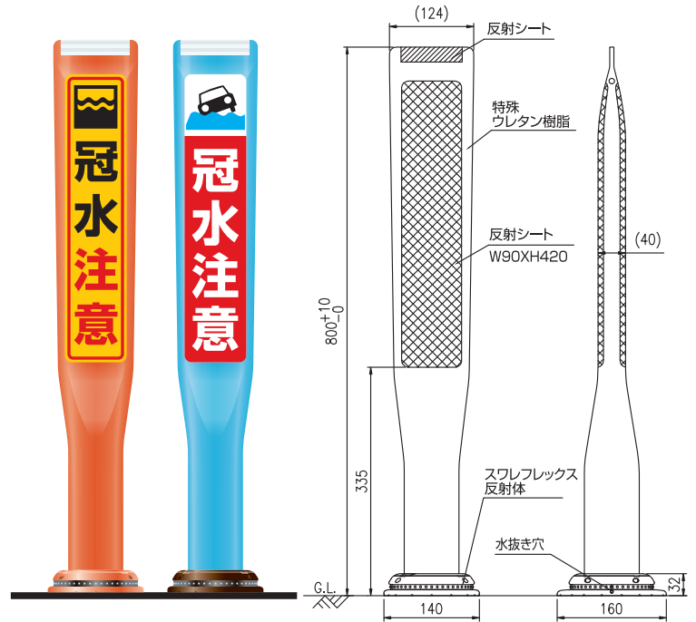
● 製品図
