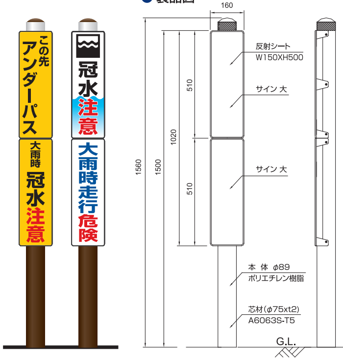
● 製品図
